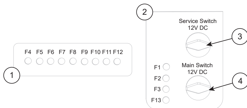
Figur 8.1 Yamarin 63 DC/BR huvudströmbrytare och säkringspanel
