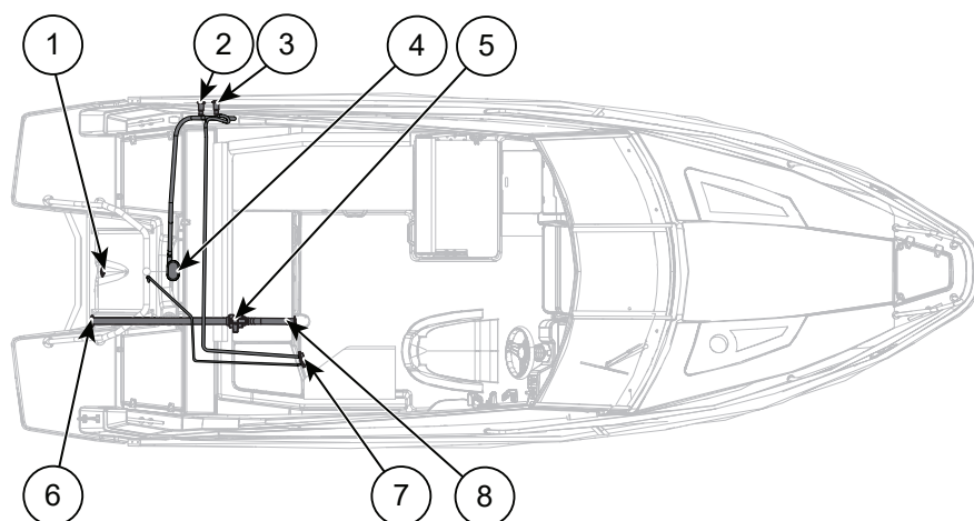
Figur 9.1 Yamarin 63 DC länspumpar och dränering
